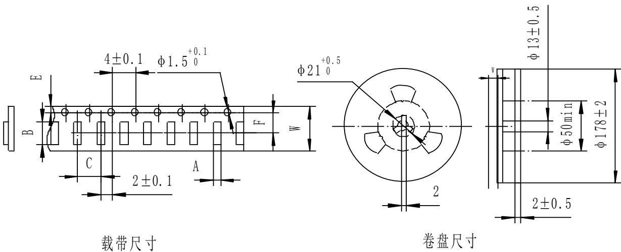
图 3 编带尺寸
